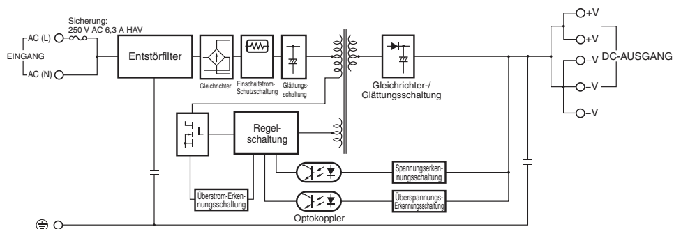
S8VK-C06024 (60 W)
