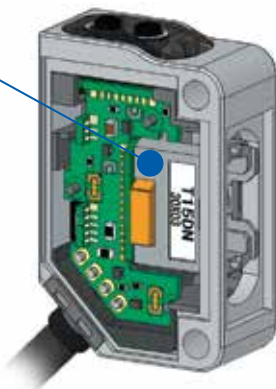
Interner Aufbau
