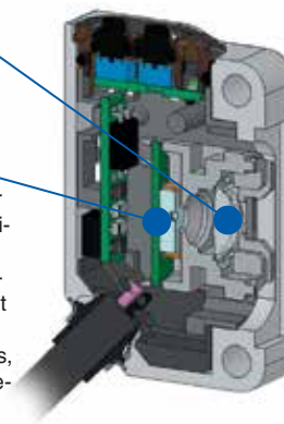
Querschnitt
