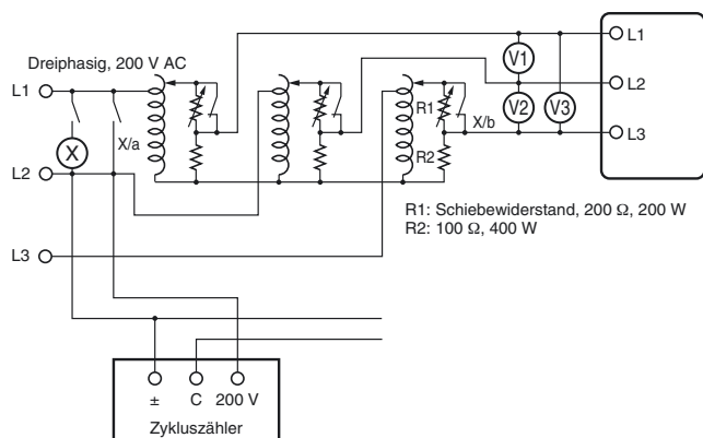
Anschlussplan 2
