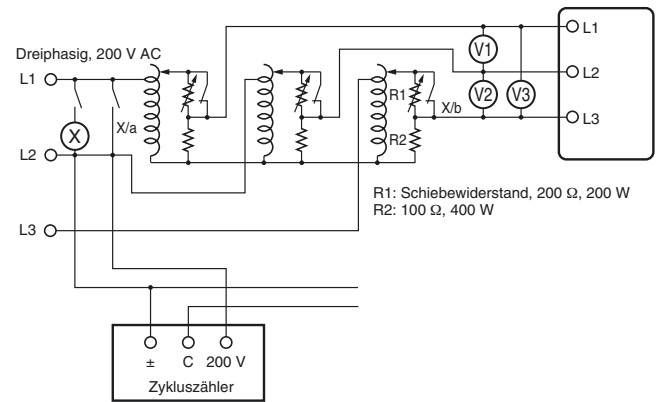
Anschlussplan 2
