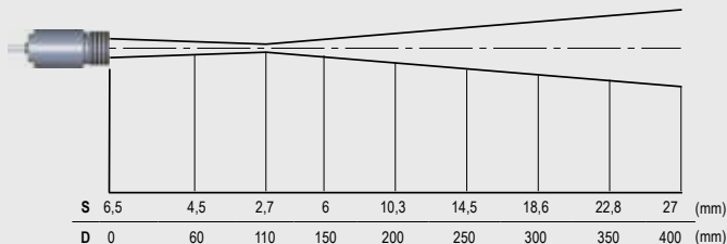
Optik CF, D:S = 40:1
