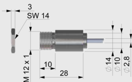
Abmessungen CSmicro
