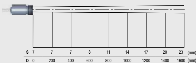
Optik SF, D:S = 75:1
