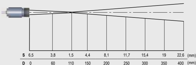
Optik CF, D:S = 75:1
