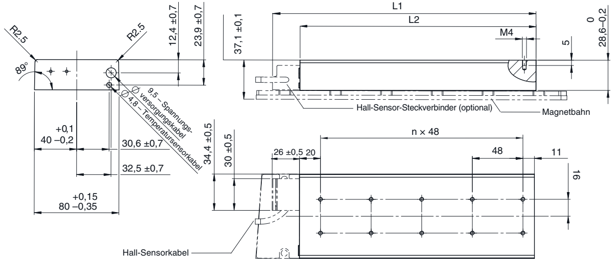
Abmessungen Motorwicklung mit Magnetbahn und Hall-Sensor (optional)
