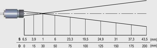
Optik CSmicro 3MH CF1, D:S = 33:1 (Fernfeld 4:1)
