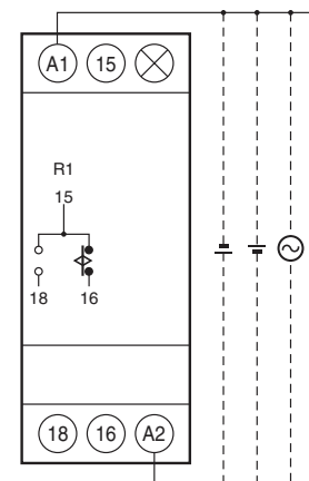
(DIN-Schaltbild)
