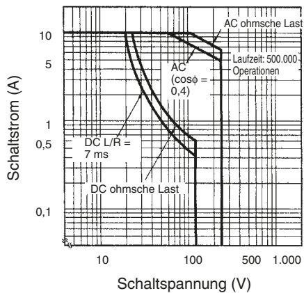
Maximale Schaltleistung
