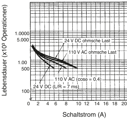
Lebensdauer
