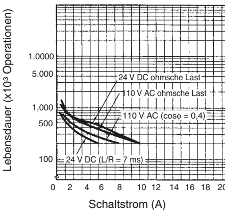
Lebensdauer
