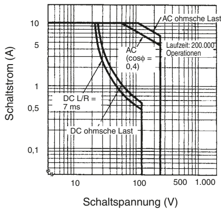
Maximale Schaltleistung
