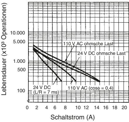
Lebensdauer
