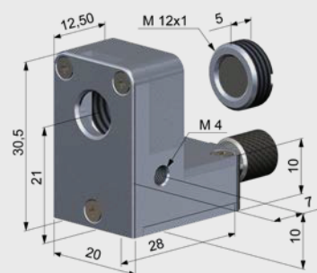
Freiblasvorsatz mit integrierter CF-Vorsatzlinse (ACCTAPLCF)
