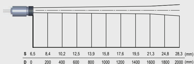
CTi 2MH/2MH1 SF, D:S = 75:1
